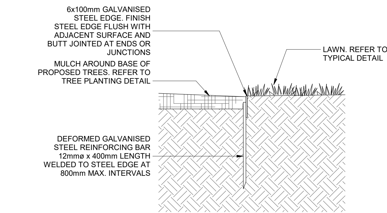
4 SE - STEEL EDGE SECTION DETAIL 1 : 10
