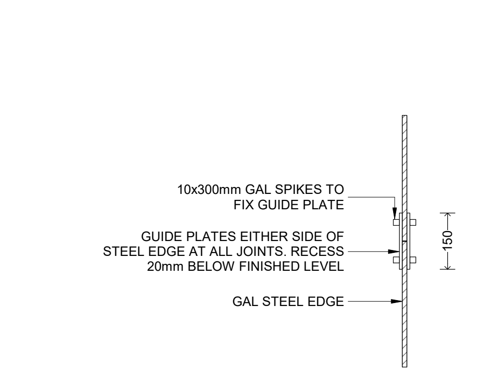
3 SE - STEEL EDGE JOIN DETAIL PLAN 1 : 10
